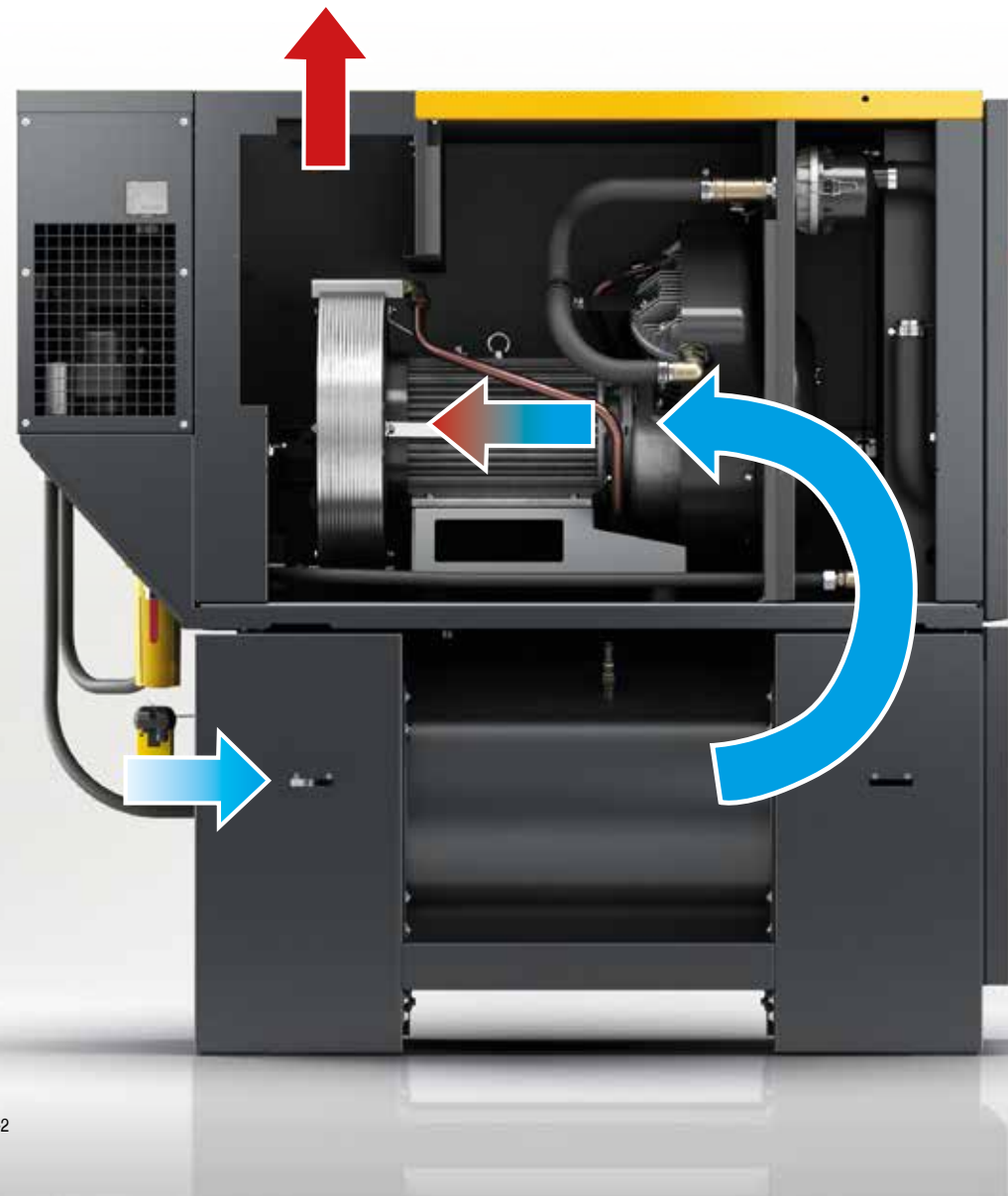
Abb.: AIRBOX 1000-2
