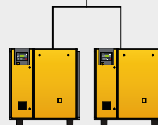
Connexion des compresseurs équipés du SIGMA CONTROL ; connexion à des stations par réseau Profibus (remplacement du SIGMA AIR MANAGER 1)
